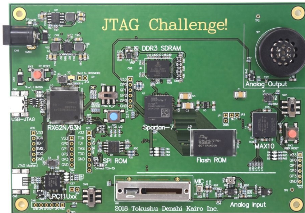
写真 わざと設計ミスが作りこまれた「JTAGチャレンジ基板」
