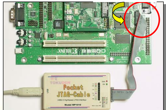
リボンケーブルで接続
