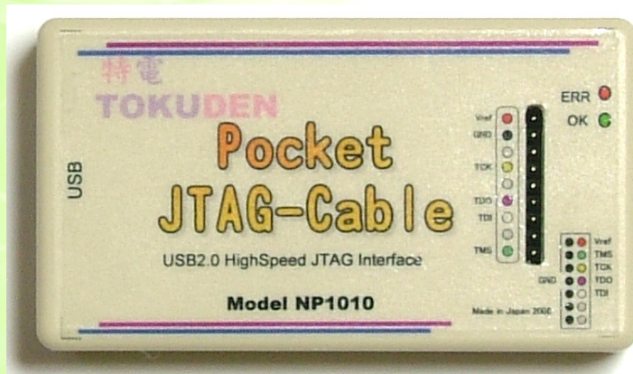
フライリードワイヤーで接続
